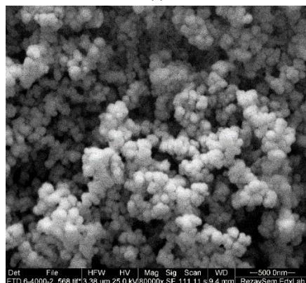
شکل ۱- تصاویر میکروسکوپ الکترونی روبشی؛ (الف) نمونه سنتز شده، (ب) پس از آزمون برون تنی
